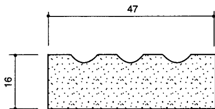
Art.Nr. 70.020.11 Listwa ozdobna
