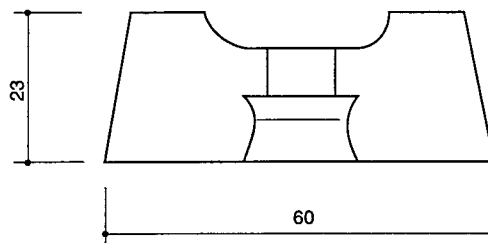
Art.Nr. 70.116.11 Listwa ozdobna
