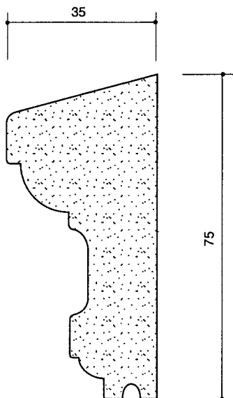
Art.Nr. 70.150.11 Listwa ozdobna
