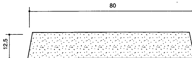
Art.Nr. 70.116.11 Listwa ozdobna
