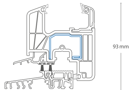
Bezbarierowy próg balkonowy / Wys. 20 mm / Rys.: 1:2,5
