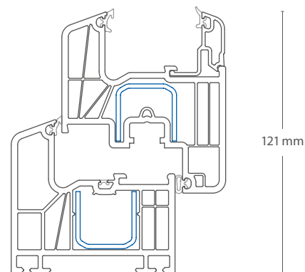
Prestige z uszczelką przylgową (AD) Rys.: 1:2,5
